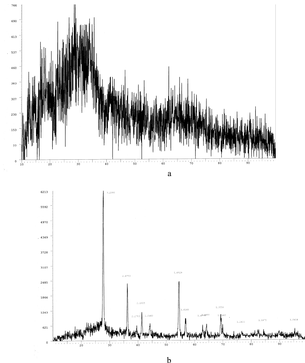
Fig. 4. XRD results. a) sample 4(32% TiO_2 ). b) sample 5(32% TiO_2 ).
